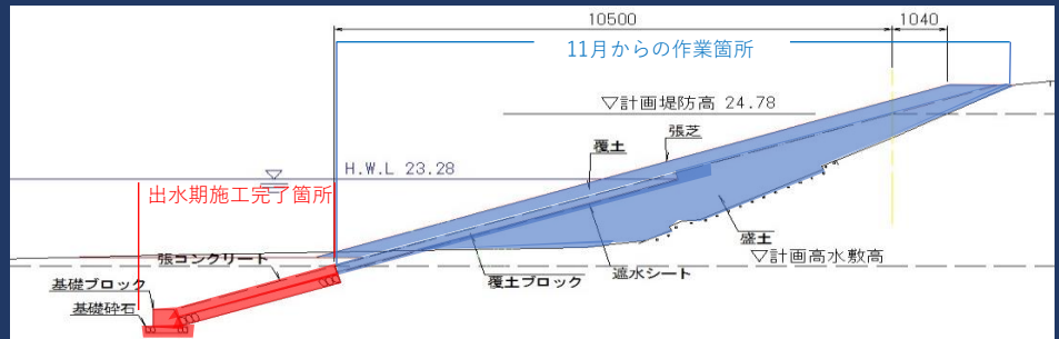
施工状況
