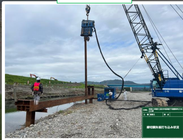
鋼矢板打込み状況
